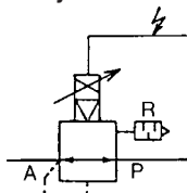
JIS Symbol
