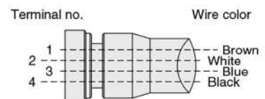
Wiring
